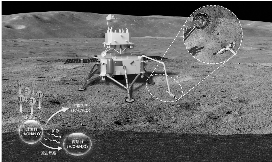
嫦娥五号月壤揭示太阳风为月球带来可利用的水。这是太阳风氢的注入、保存与扩散丢失模型图(2022年11月23日绘制)。
