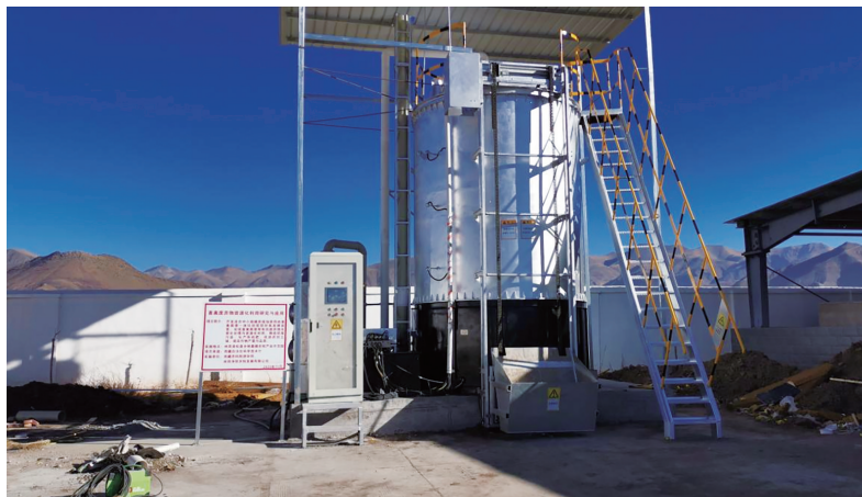
图由自治区农科院资环所提供 畜禽粪便发酵处理塔。
