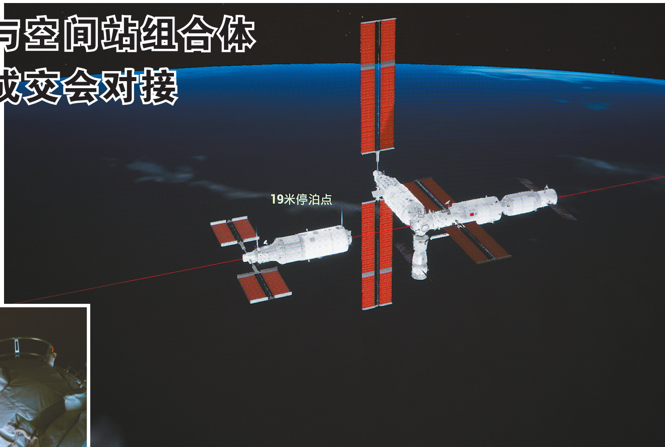
▲梦天实验舱从19米停泊点向天和核心舱前向端口靠近的模拟图像。 ▲梦天实验舱对接锁紧完成。
